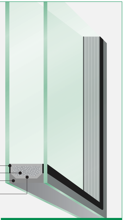
Schematischer Aufbau von Zweifach-Isolierglas
